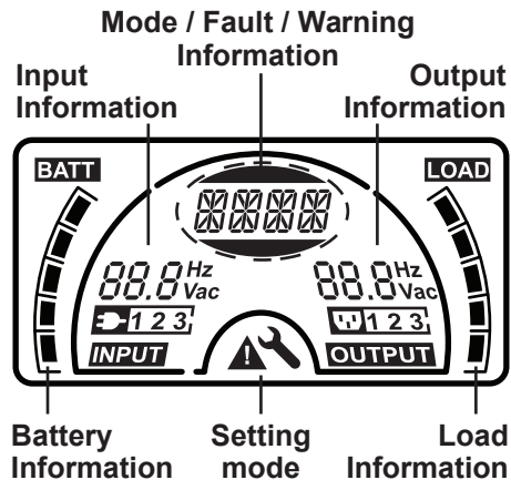
Рисунок 4.2 LCD дисплей
