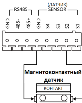
Рисунок 5-18 Подключение магнитоcontactного датчика для моделей DS-KD8102-V/DS-KD8002-VM (2)
